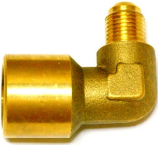
ITEM NUMBER : 134 – DİRSEK SIZES (ÖLÇÜLER): 1/2 NPT – 1/4 HAVŞA
